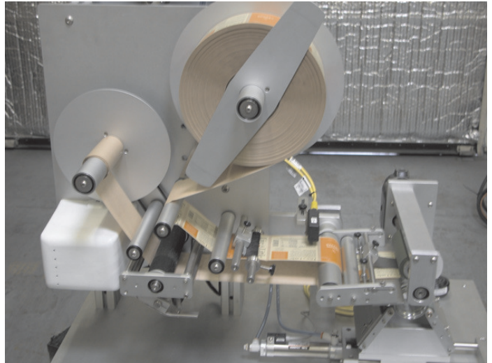
WRAP APPLICATOR
